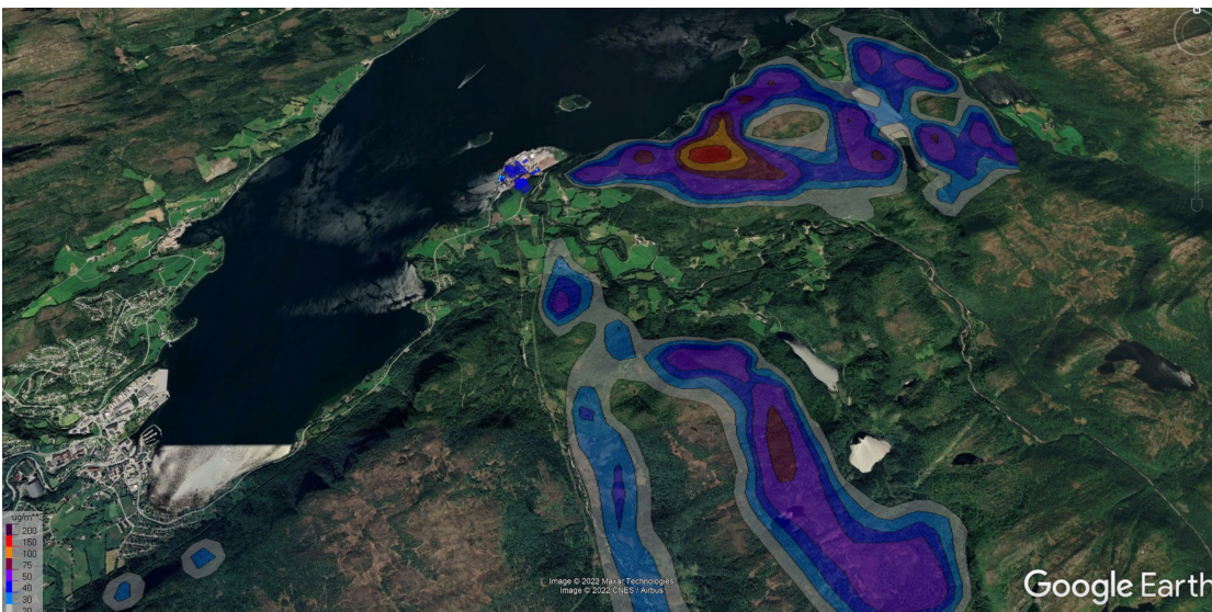
Figur 17 Høyeste døgnmiddelbidrag av svevestøv (µg/m 3 ). Nødskorstein Ovn 9. Utslipp kl. 7-8
