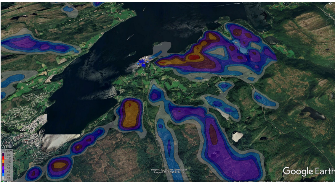
Figur 18 Høyeste døgnmiddelbidrag av svevestøv (µg/m 3 ). Nødskorstein Ovn 9. Utslipp kl. 7-10
