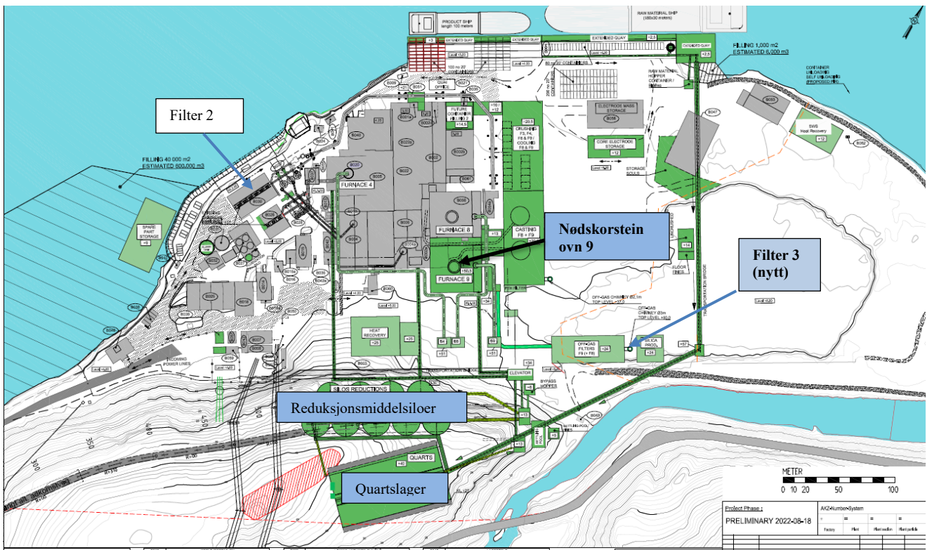
Figur 5 Lokalisering av filtre, nødskorstein ovn 9 samt quartslager og reduksjonsmiddelsiloer
