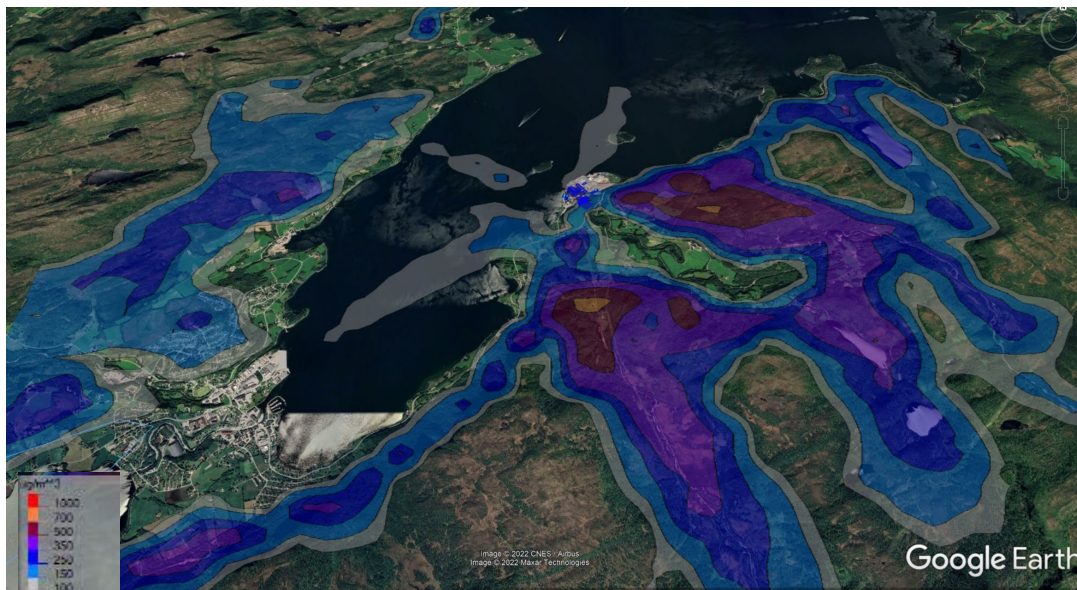
Figur 9 Høyeste timemiddelbidrag av SO 2 (µg/m 3 )
