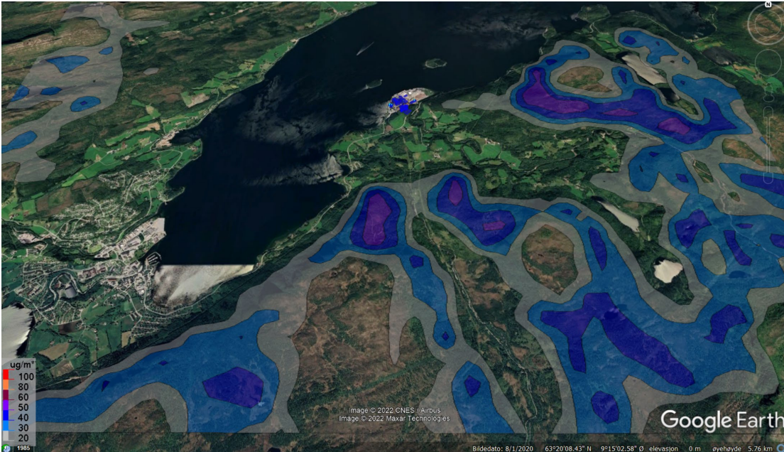
Figur 14 Høyeste bakkekonsentrasjonsbidrag av NO 2 (µg/m 3 , timemiddel)
