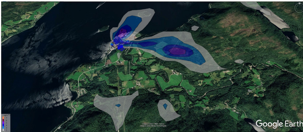
Figur 12 Høyeste døgnmiddelbidrag av svevestøv ( \mu\text{g}/\text{m}^3 )
