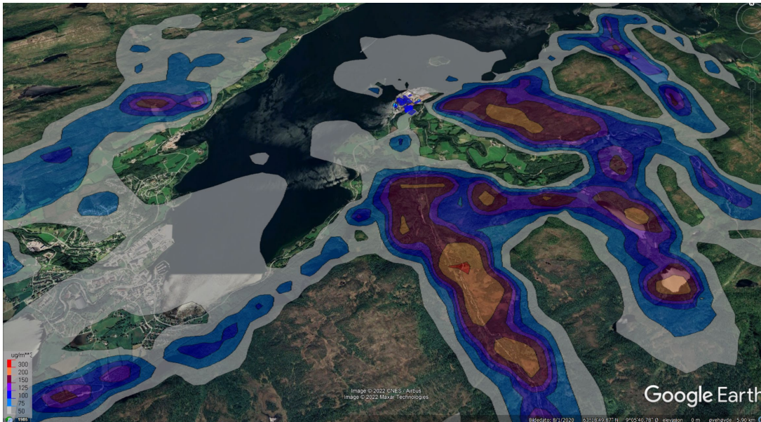
Figur 6 Høyeste bakkekonsentrasjonsbidrag av NO 2 (µg/m 3 , timemiddel).
